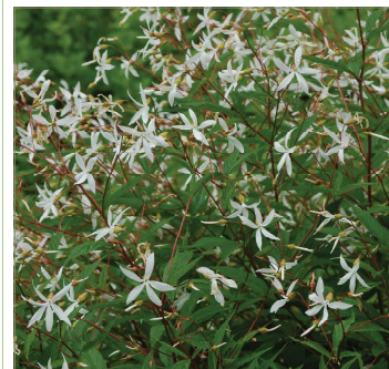
Porteranthus trifolius
